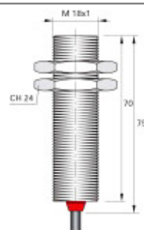
Dimensioni in mm
